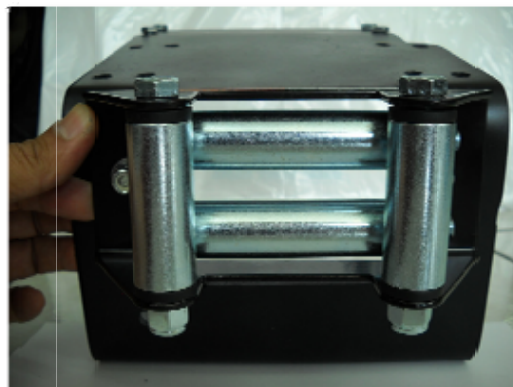
Fig. 3.4 Vista Frontal
